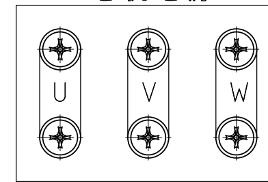
Motor 电机电源
